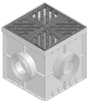
Recyfix punktavløp: Mål: 30x30x30cm Teknisk tegning. DoP/Ytelseserklæring. Installering. Produktdatablad.
