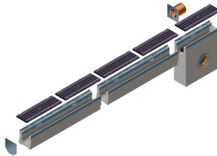
Faserfix sandfang: Teknisk tegning.
